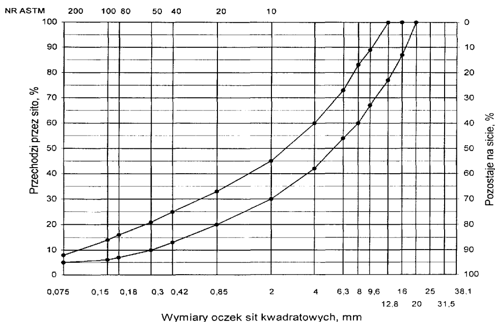
Rys. 1. Krzywe graniczne uziarnienia mieszanki mineralnej BA od 0 do 16 mm do warstwy wyrównawczej nawierzchni drogi.
