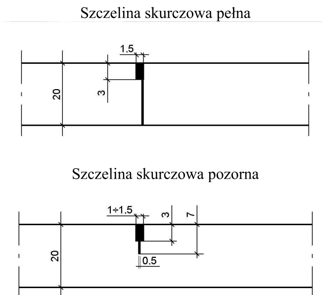
Rys. 1.1. Przykłady konstrukcji szczelin w podbudowie z betonu cementowego (wymiar w cm)
